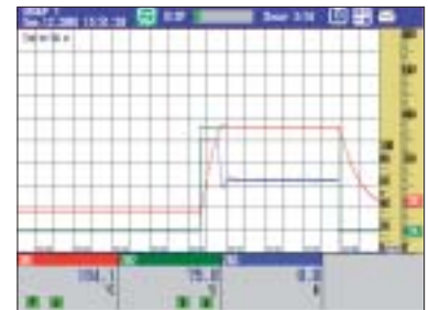
Дисплей тренда Этот дисплей может отображать кривые PV, SP, и OUT контура управления, а также кривые обычных измерительных каналов.
